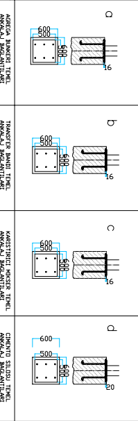
BETON SANTRALI ANKALAJLARININ TEKNİK RESİMLERİ
